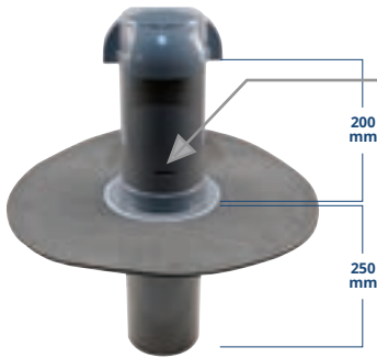
Sanitärlüfter KW mit Kondenswasser-Abscheider
