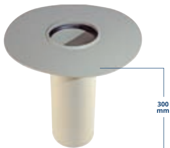
Unterteil RS mit Dichtung zur Rückstausicherung
