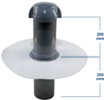
Sanitärlüfter mit abnehmbarer Wetterkappe
